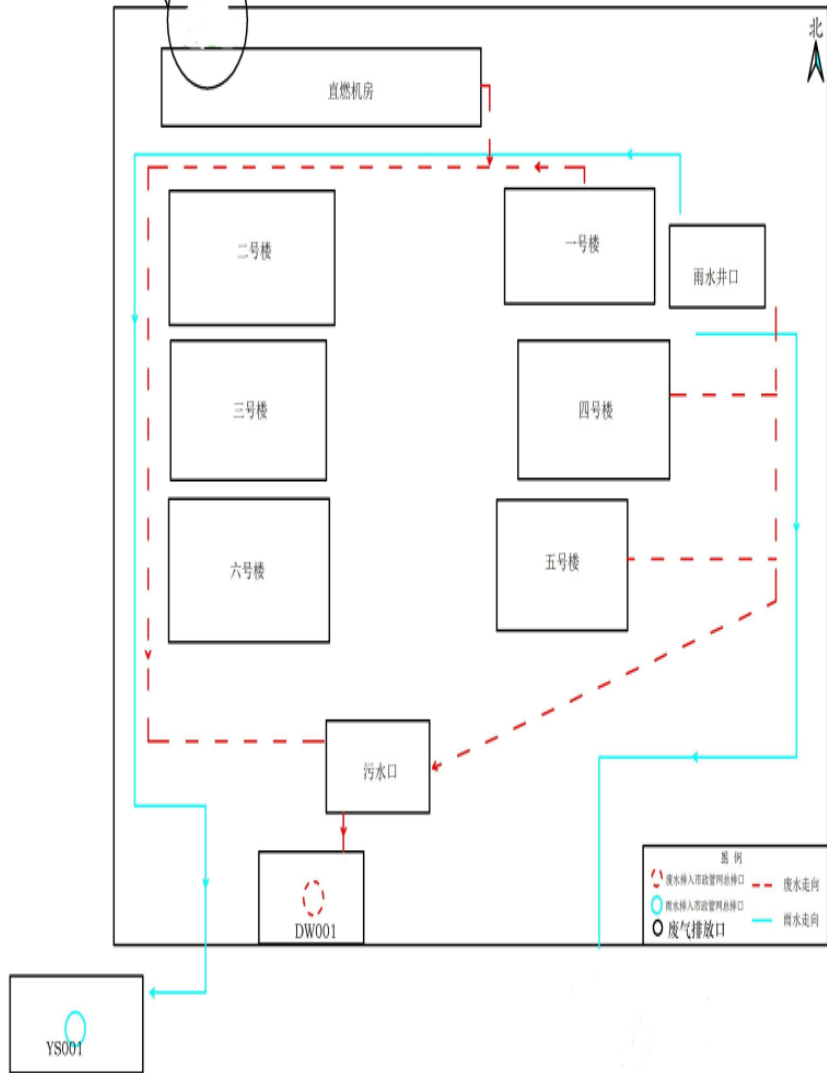
三区生产厂区总平面布置图
